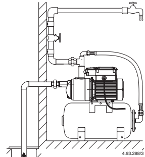
Fig. 2 Funzionamento in aspirazione Suction lift operation Saugbetrieb Fonctionnement en aspiration Funcionamiento en aspiración Sugande funkcion Zuigsituatie Θέση λειτουργίας με κάθετη αναρρόφηση Работа выше уровня жидкости 负吸水头工作
